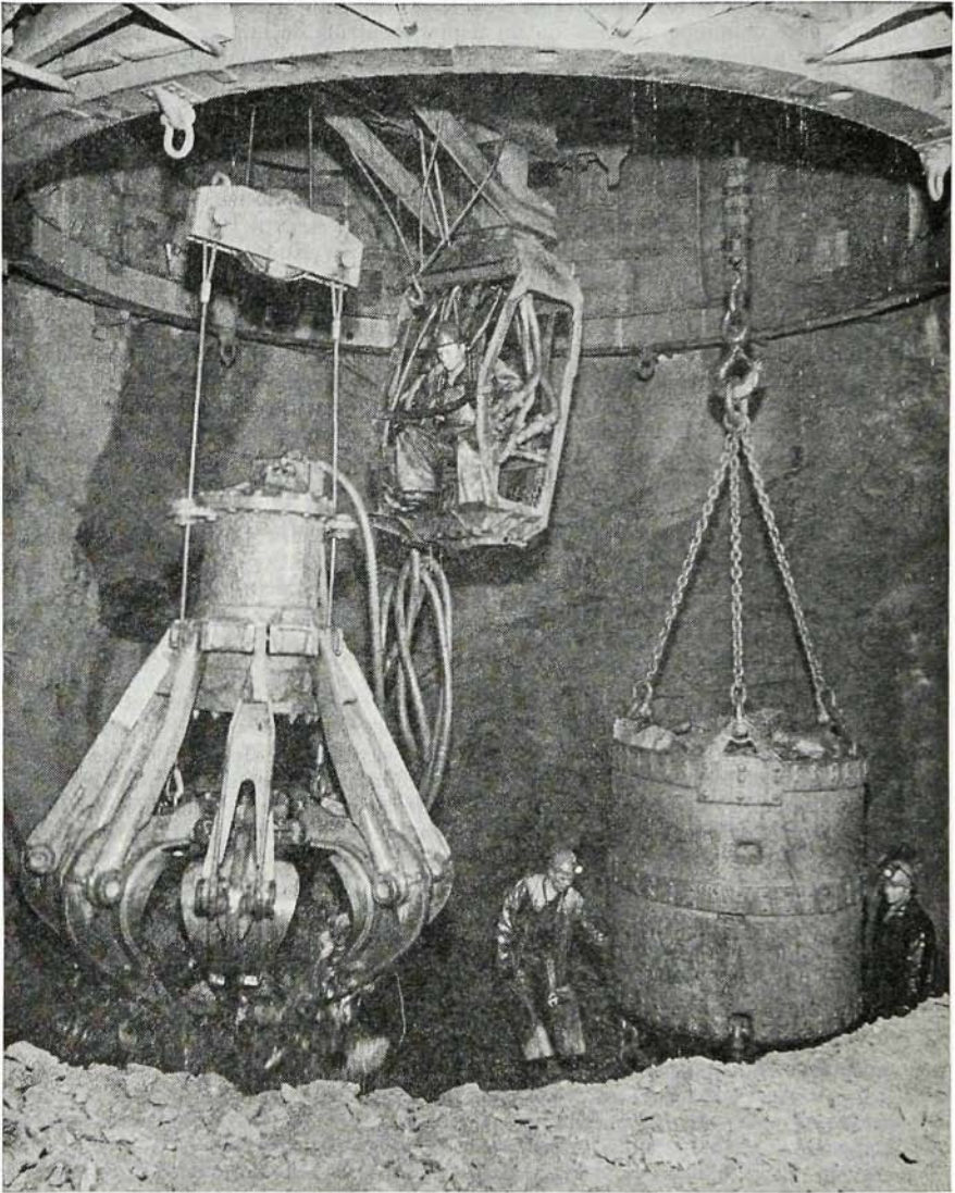
Le puits n° 9 de la mine Creighton de l'International Nickel près de Sudbury (Ont.) atteindra sa profondeur maximum de 7,150 pieds au début de 1969. C'est un des deux puits en voie d'être foncés aux mines actives de la société. Cinq nouvelles mines dans la région de Sudbury et trois autres près de Thompson (Man.), s'ajouteront aux usines de traitement agrandies pour augmenter la capacité théorique de production canadienne de nickel de la société de 100 à 150 millions de livres d'ici 1970.
